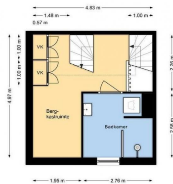
Rijksbes 79 2e Verdieping Hoogte 2.47/ 5.70m
