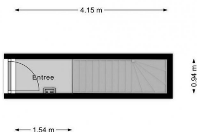
MEIDOORNSTRAAT 61 1e Verdieping Hoogte 2.72m
