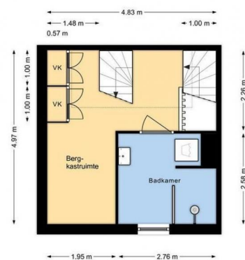
Rijksbes 79 2e Verdieping Hoogte 2.47/ 5.70m
